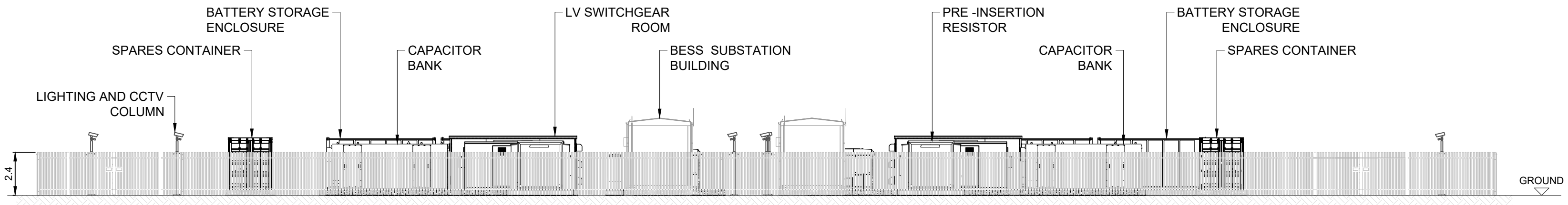
PLAN VIEW SCALE 1:1,000
